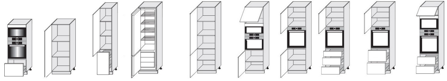
D5AM/60/154 600/1540/565 D5AA/60/154 600/1540/565 2D14K/40 400/2070/565 CARGO D14/DL/60/207 600/2070/565 D14/DP/60/207 600/2070/565 D14/RU/60/207 600/2070/565 D14/RU/2D 600/2070/565 D14/RU/3M 600/2070/565 D14/RU/3A 600/2070/565 D14/RU/2M 356 600/2070/565 D14/RU/2A 284 600/2070/565 D14/RU/2M 284 600/2070/565
