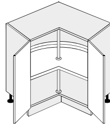
D12/90 KOSZ 840/820/840
