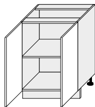
D11/60 600/820/500
