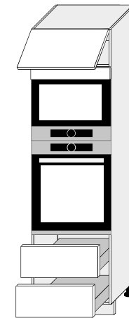
D14/RU/2M 284* 600/2070/565
