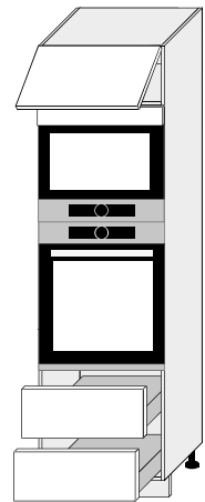
D14/RU/2E 284* 600/2070/565
