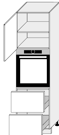
D14/RU/2M 356* 600/2070/565
