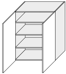
W4/80* 800/960/325
