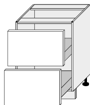
D2E/60* 600/820/500
