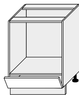
D11K/60 600/820/500
