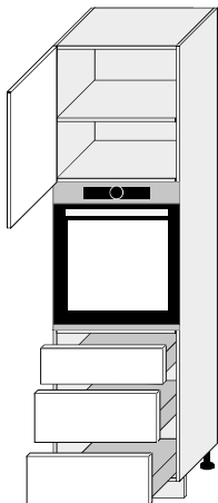
D14/RU/3M* 600/2070/565
