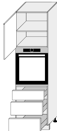
D14/RU/3E* 600/2070/565
