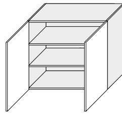
W3/90 900/720/325* 900/720/300**
