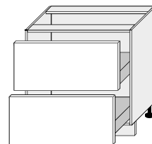
D2E/80* 800/820/500
