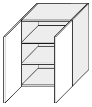
W3/60 600/720/325* 600/720/300**
