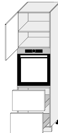
D14/RU/2E 356* 600/2070/565
